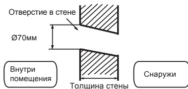
Стенное отверстие в разрезе
